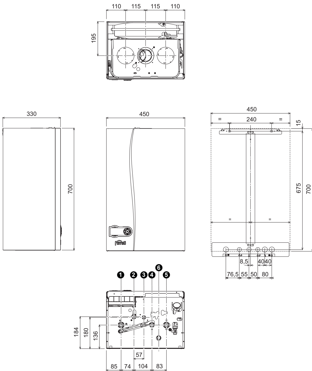
мал. 30 - Розміри та під'єднання
