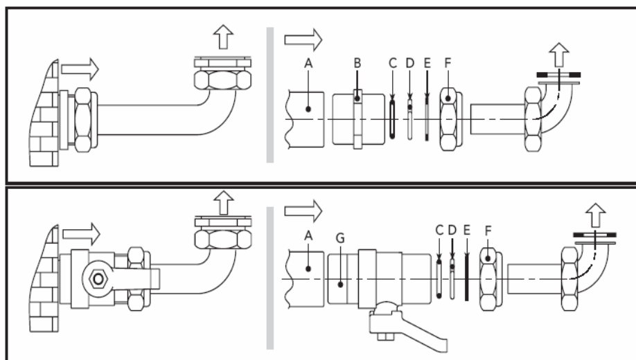
мал. 17 - Набір для підключення
