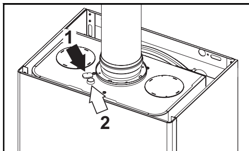
мал. 29 - Аналіз відпрацьованих газів
