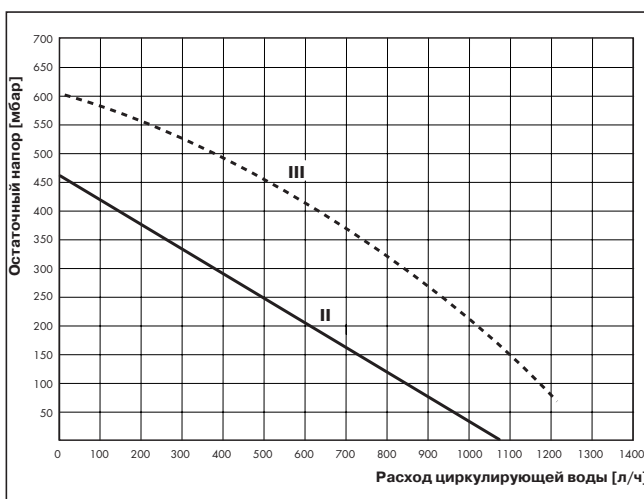
Рис. 6.4 Характеристика насоса
