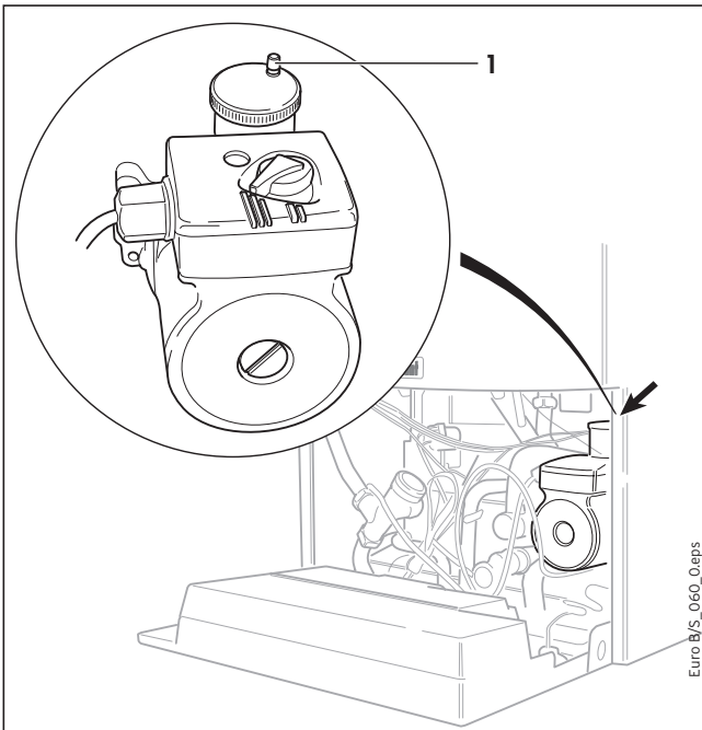
Рис. 3.16 Автоматический воздухоотводчик
