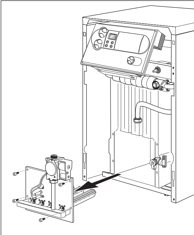
Slika 7.1 Demontaža plamenika
