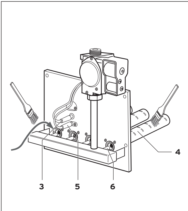
Slika 7.3 Čišćenje plamenika
