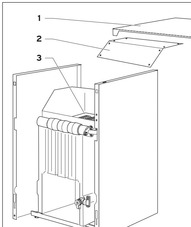
Рис. 7.2 Чистка теплообменника
