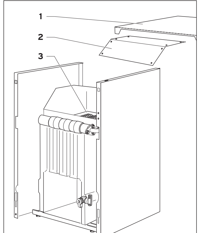
Slika 7.2 Čišćenje izmjenjivača topline
