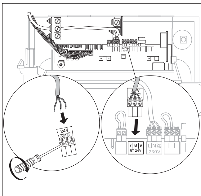
Sl. 4.8 Priklučiti regulator na stezaljke 7-8-9
