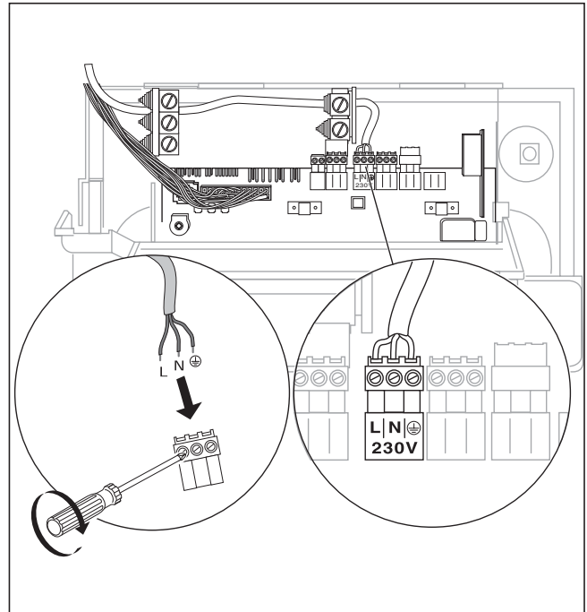
Sl. 4.5 Priključitev dovoda elektrike
