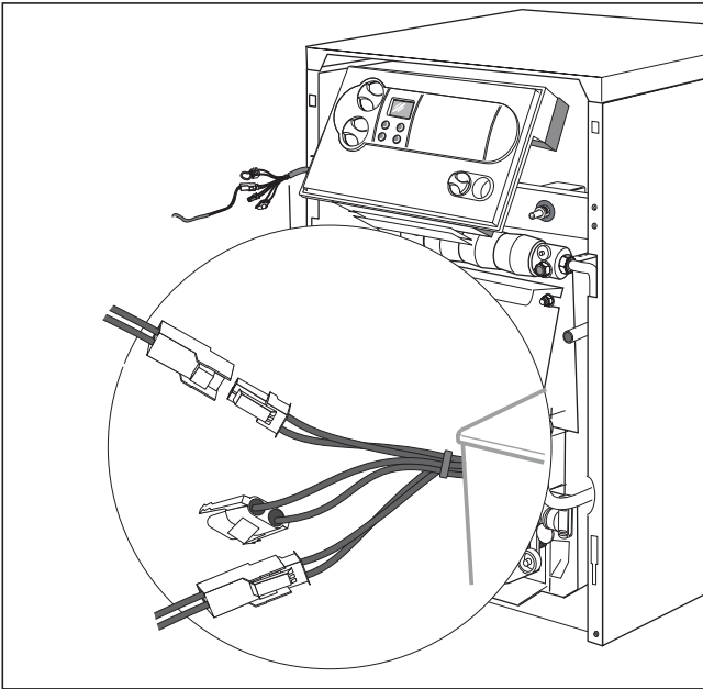
Рис. 4.7 Подключение датчиков
