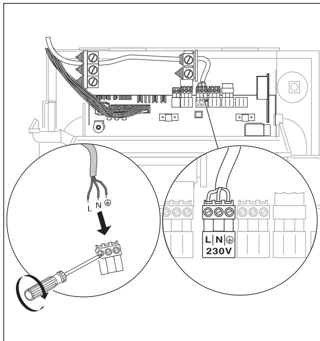
Slika 4.5: Priklučivanje mrežnog voda
