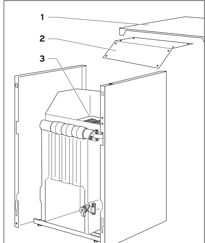
Sl. 7.2 Čiščenje toplotnega izmenjevalnika
