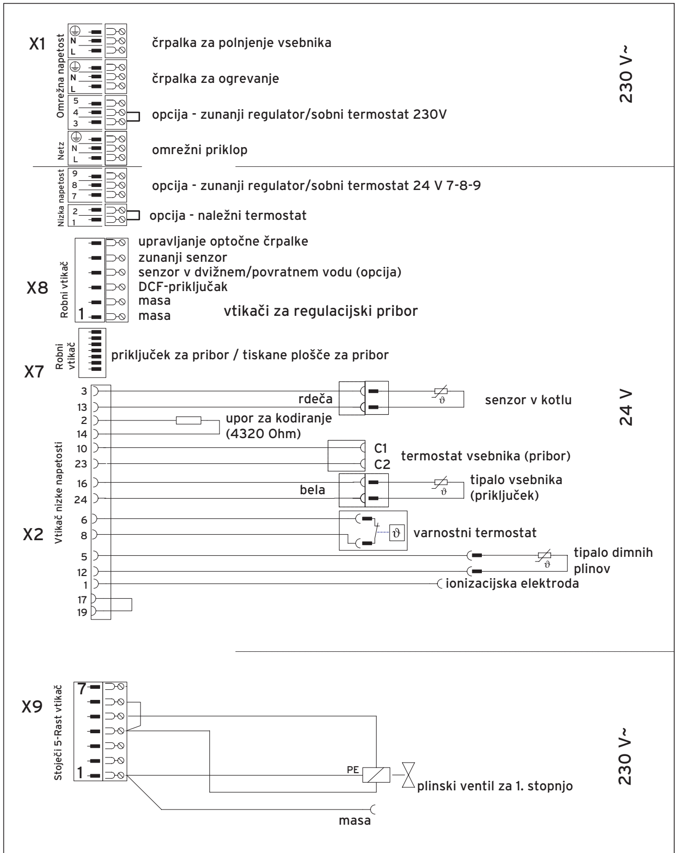
Sl. 4.6 Električni priključki atmoVIT
