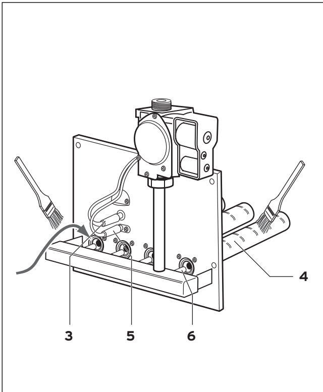
Fig. 7.3 Curățarea arzătorului
