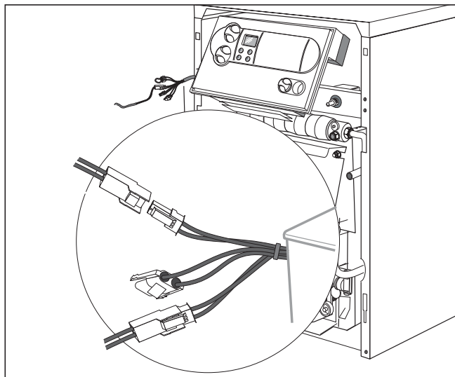
Slika 4.7: Priklučivanje senzora
