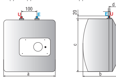
МОДЕЛЬ ДЛЯ МОНТАЖА ПОД РАКОВИНОЙ
