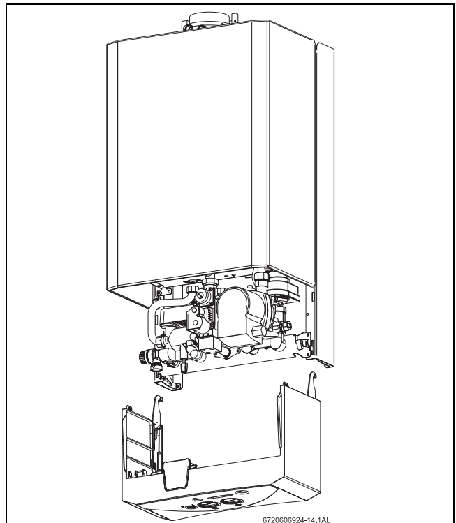
Рис. 9 Демонтаж розподільної скриньки
