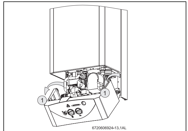
Рис. 21 Сервісна позиція
