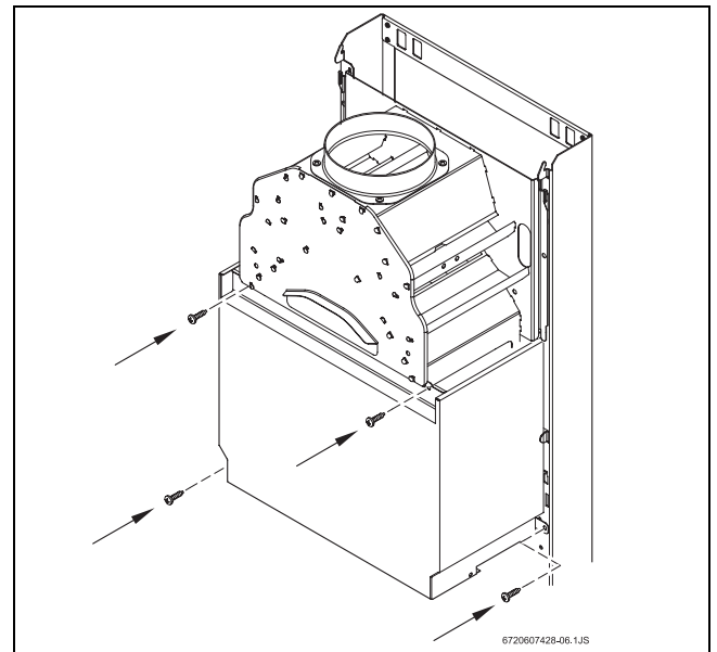
Рис. 23 Захисна кришка
