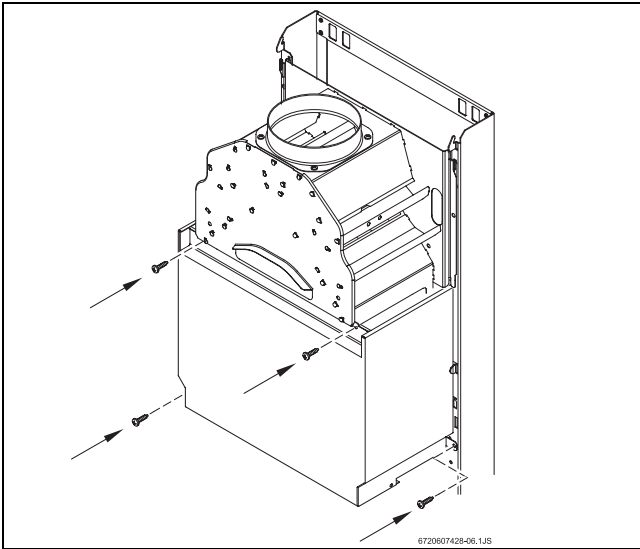
Рис. 24 Захисна кришка
