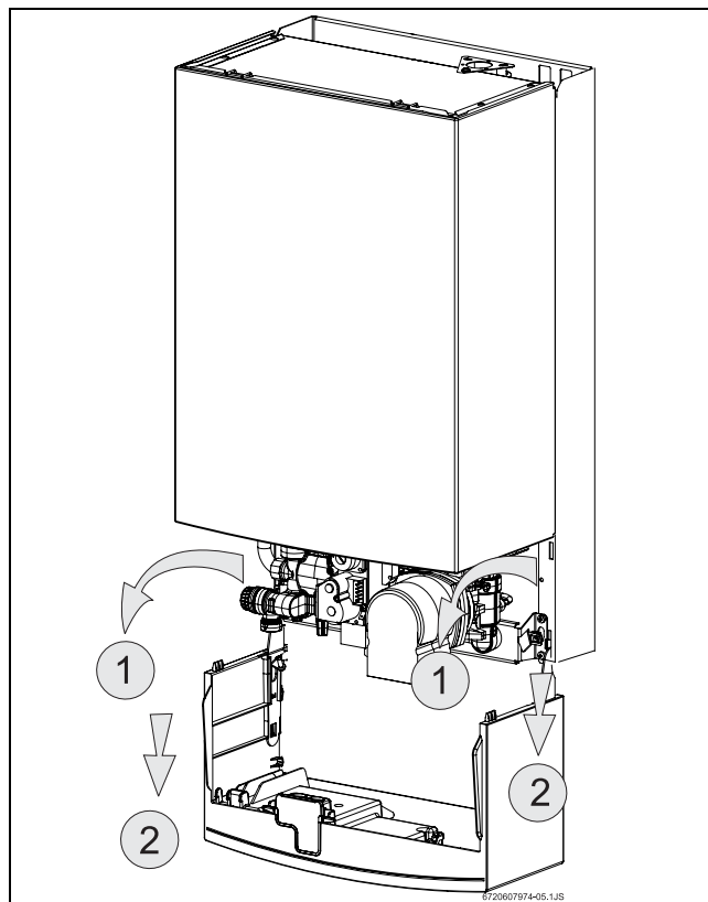
Рис. 8 Блок у положенні технічного обслуговування, що забезпечує доступ до вузлів водяної арматури та електронної системи.
