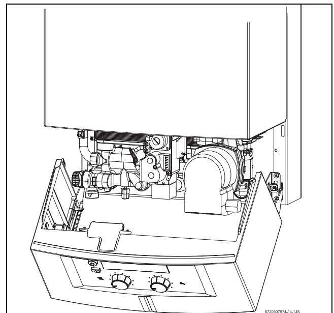
Рис. 22 Блок у сервісному положенні
