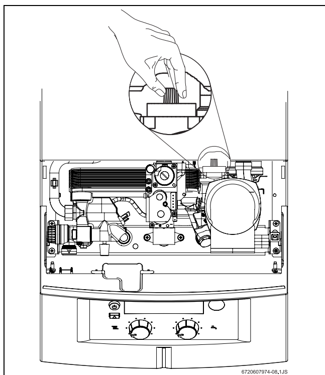
Рис. 12 Відкриття спускного клапана
