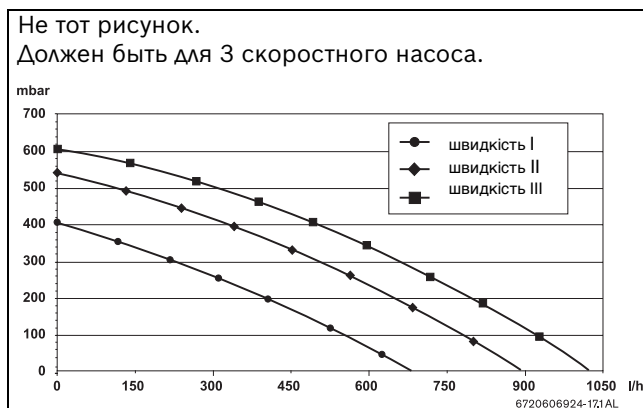
Рис. 4 Криві характеристик насосу
