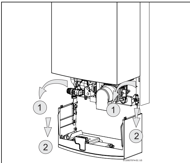
Рис. 26 Блок у положенні технічного обслуговування, що забезпечує доступ до вузлів водяної арматури та електронної системи
