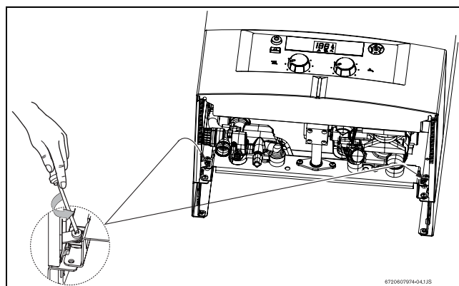
Рис. 7 Кріпильні гвинти
