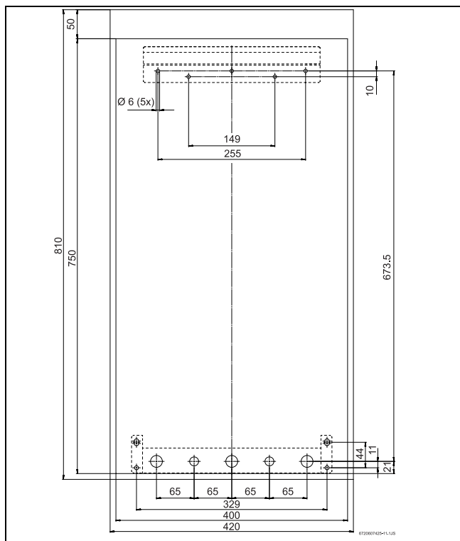
Рис. 6 Кріпильна рейка та монтажна планка
