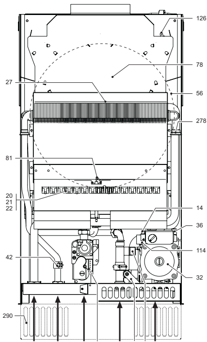
мал. 8 - Загальний вигляд DOMproject C 32
