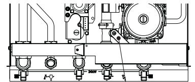
мал. 3 - Кран для заправлення
