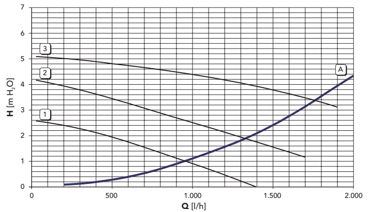
мал. 9 - Утрати напору / тиску циркуляційних насосів DOMproject C 24
