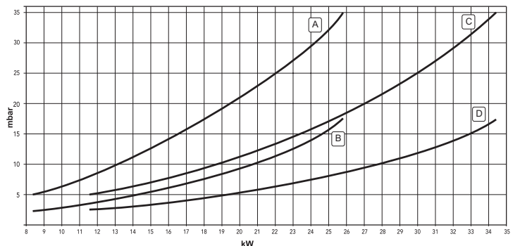
мал. 11 - Діафрагма тиску - потужність
