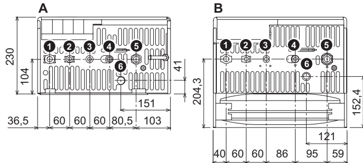
мал. 4 - Гідротехнічні підключення
