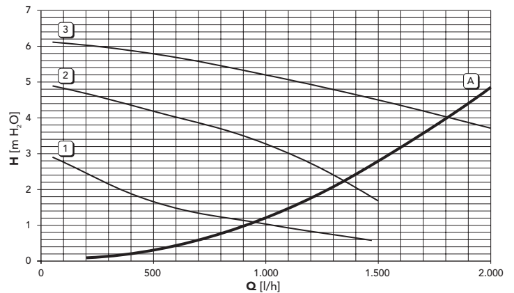
мал. 10 - Утрати напору / тиску циркуляційних насосів DOMproject C 32
