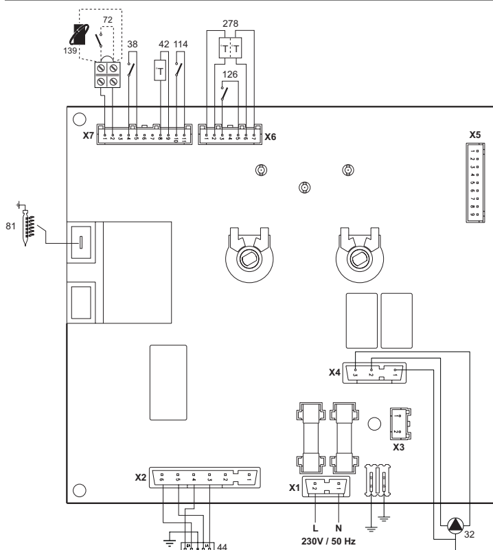
mal. 12 - Електрична схема
