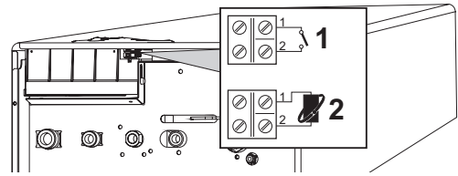
мал. 5 - Доступ до клемної коробки
