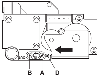
мал. 6 - Газовий клапан
