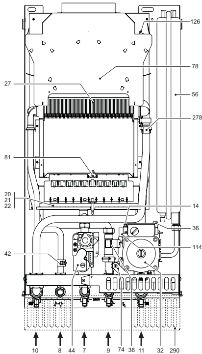
мал. 7 - Загальний вигляд DOMproject C 24
