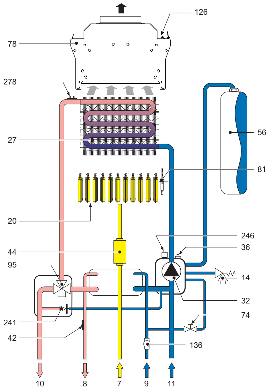
мал. 25 - Гідравлічний контур
